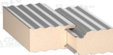
СЭНДВИЧ-ПАНЕЛИ МВУ С ЗАМКОВ S-FIX
